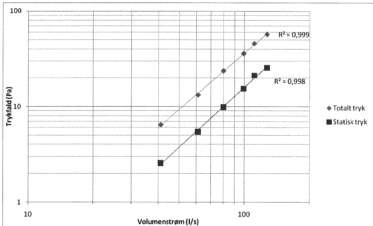
Kapacitetsdiagram: Stor hætte tilsluttet Ø160 mm rør.
