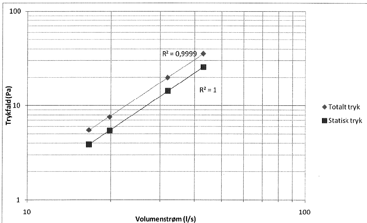
Kapacitetsdiagram: Lille hætte tilsluttet Ø125 mm rør.
